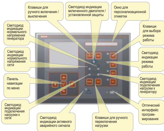
Передняя панель RGK900
