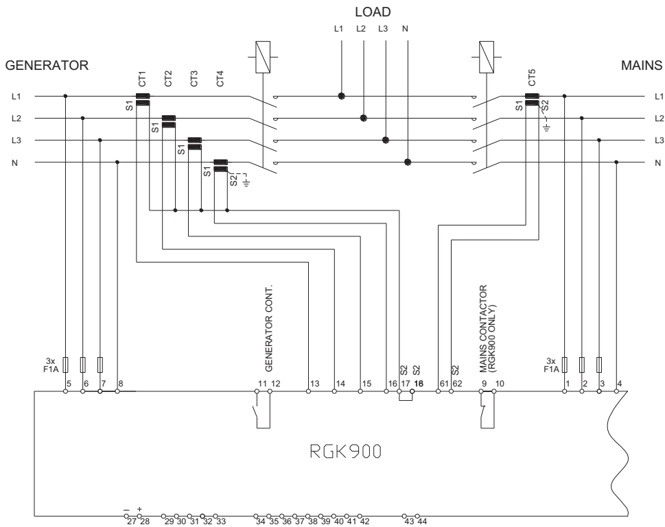
RGK900 - Типичное применение с использованием одной генераторной установки, подключенной параллельно сети RGK900 – Typical application with single genset in parallel to mains
